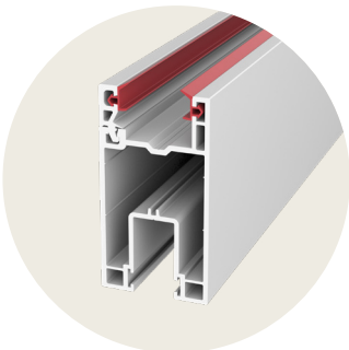
5 양면 가스켓 유럽 시스템 창호에 적용되는 가스켓 타입 창짝
