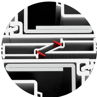
4 4중 기밀구조 여림대 부분 4중 기밀구조 적용으로 기밀성 강화
