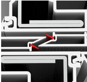
4중 기밀구조 여밈대 부분 4중 기밀구조 적용으로 기밀성 강화
